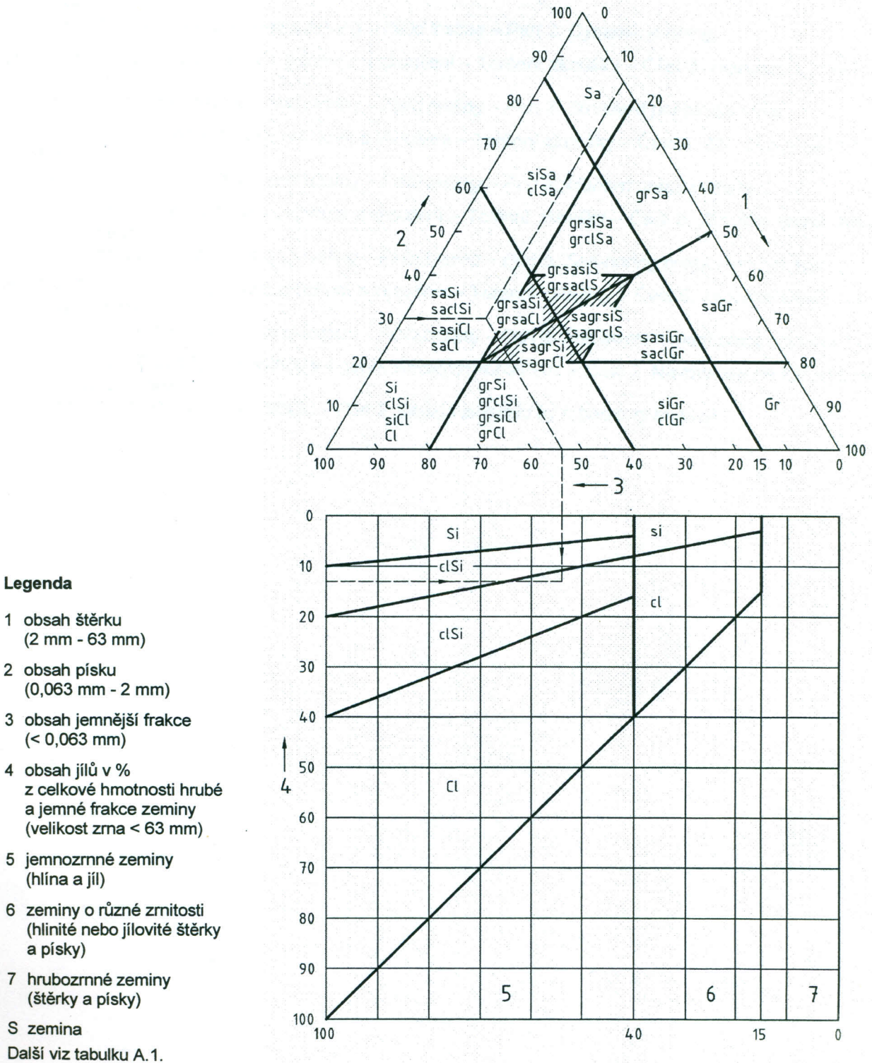
Obrázek B.1 – Zatřídování zemin pouze na základě zrnitosti
